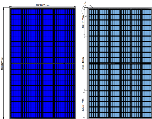
组件尺寸
